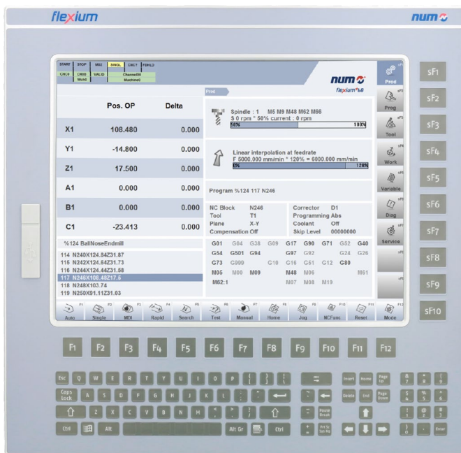
帶 22 個功能鍵和 QWERTY 鍵盤的面板
