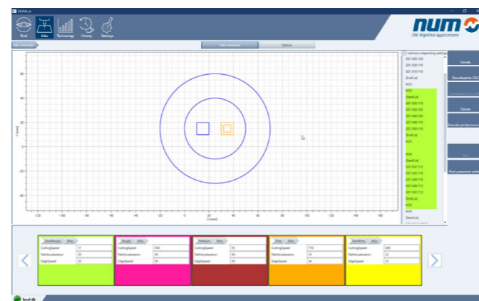
Figure 2 : Attribution de la qualité de coupe
