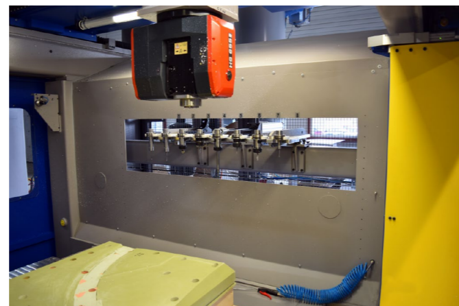
Détails de la tête RTCP et du changeur droit.
