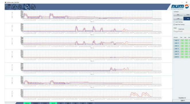
Exemple d'une machine où 7 axes sont surveillés. Bleu : valeur moyenne du courant des axes mesurés lorsque la machine est neuve et testée, Rouge : courbes des enveloppes minimales et maximales
