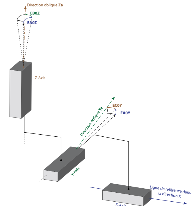
Fig.2 Ensemble d'erreurs d'orientation pour la compensation de perpendicularité d'une machine 3 axes wXYZt
