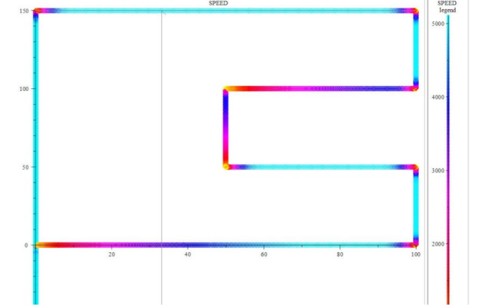
Figure 4 : Vitesse de coupe adaptative
