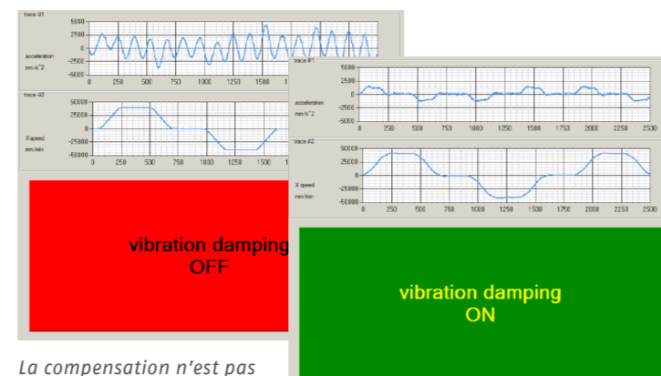
Trace # 2 : Vitesse de l'axe X, Trace #1 : Le point final vibre à sa fréquence naturelle (environ 3 Hz)
