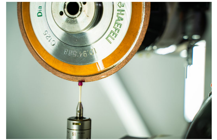
Fonction NUMROTO étendue : palpeur de meule
