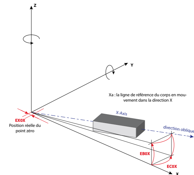
Fig.1 Erreur de position pour un axe linéaire (axe X)
