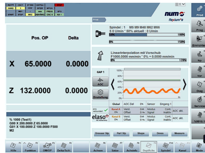
Commande NUM Flexium+ 8 avec intégration du capteur GAP
