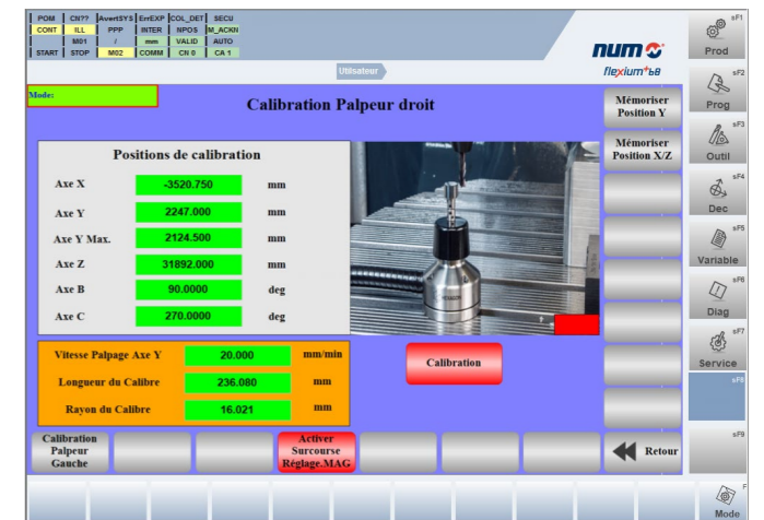
Un exemple de page d'IHM personnalisée : Calibration palpeur
