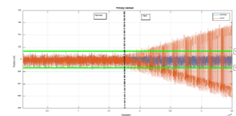
Cet exemple montre l'erreur résiduelle sur une variable surveillée ; lorsqu'une erreur se produit (côté droit), l'erreur résiduelle augmente et un avertissement est émis.
