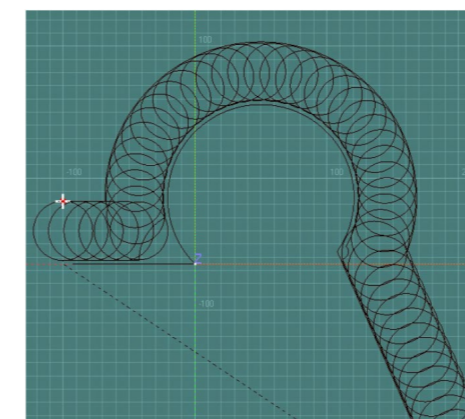
FXS0000700 Cycle de fraisage trochoïdal (G725)
