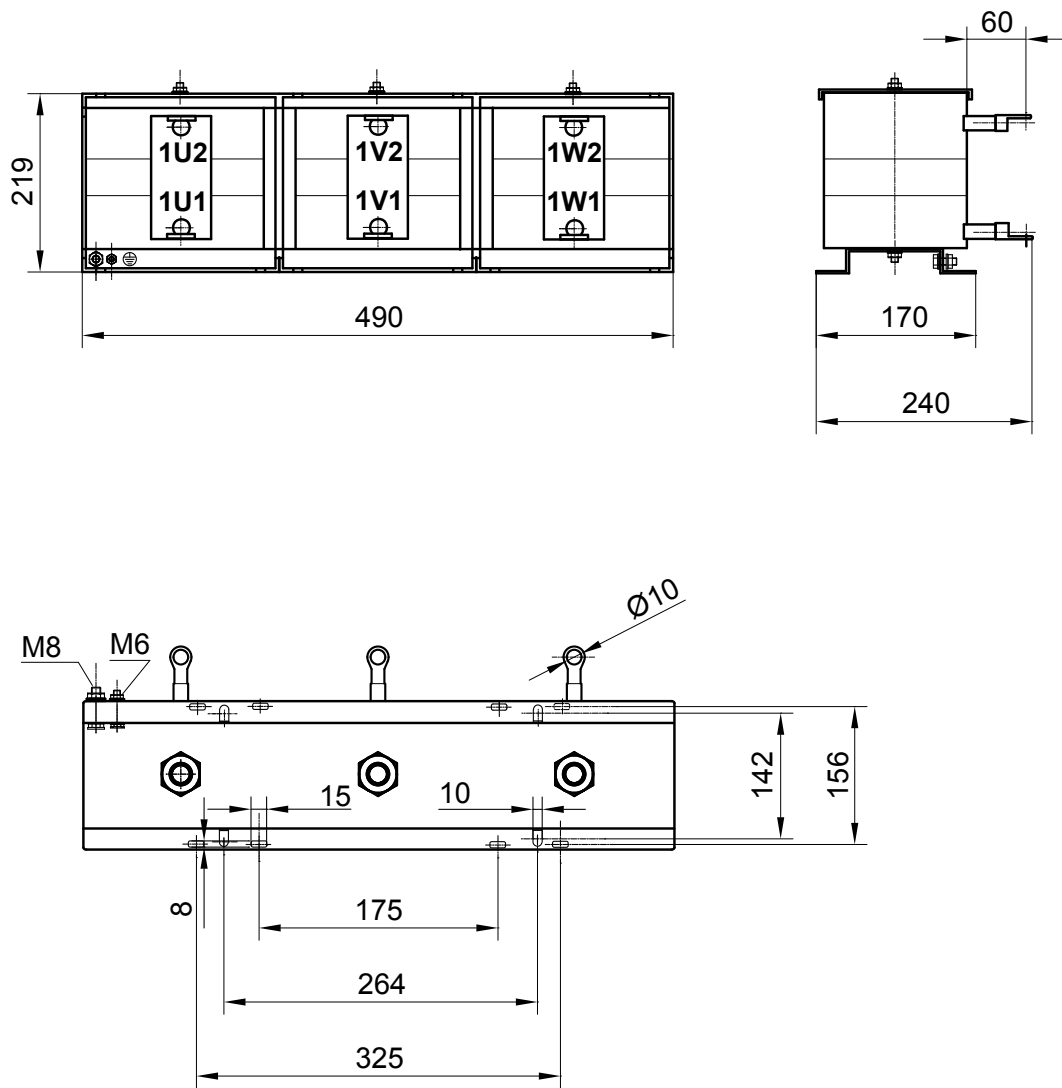
AGOIND009 - 总体尺寸
