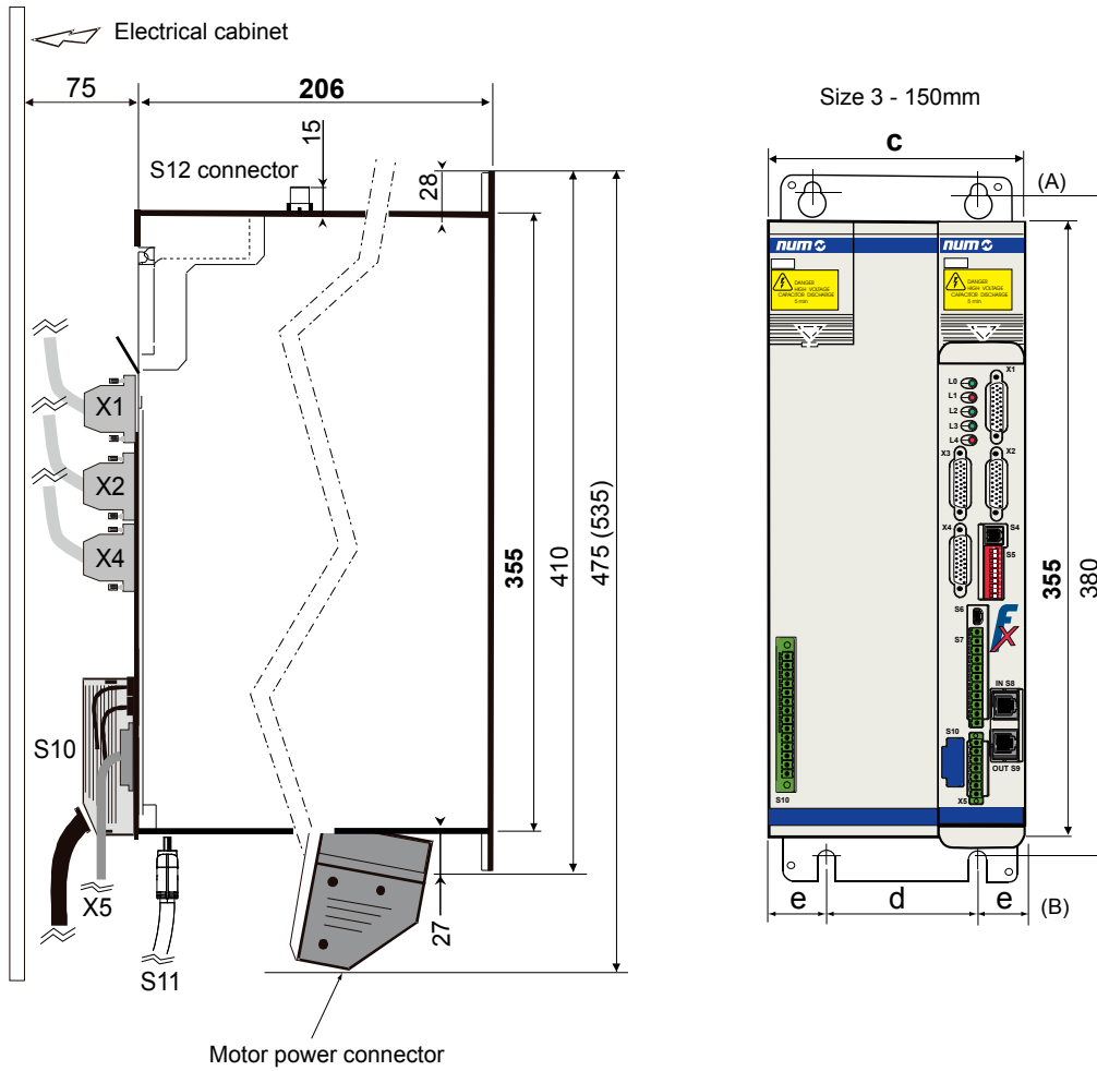
MDLUX 外形图 (尺寸 3)
