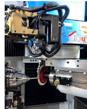
Brosse dans la machine à affûter les outils
