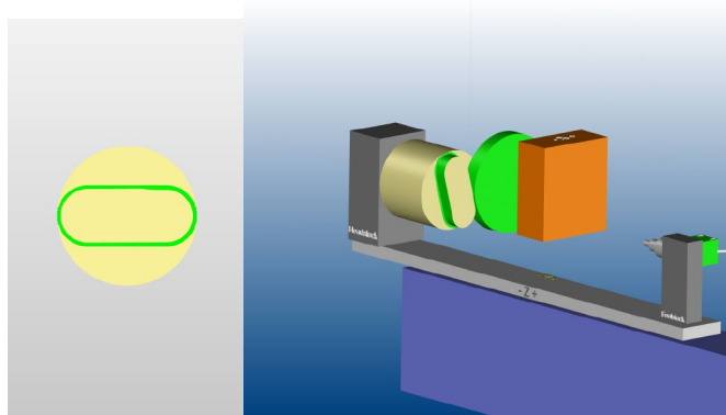
Simulazione 3D della rettifica non circolare
