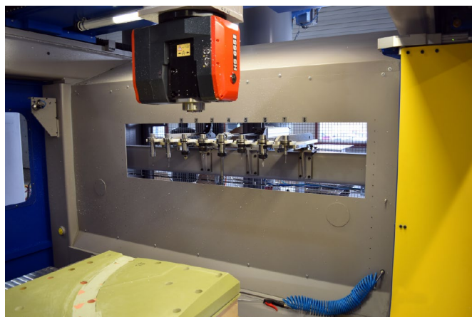
Dettagli della testa RTCP e la zona destra del cambio utensile
