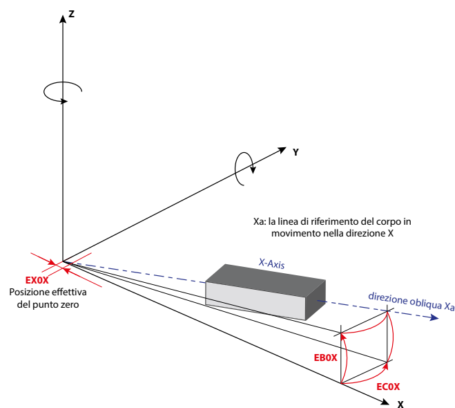
Fig.1 Errore di posizione per un asse lineare (asse X)
