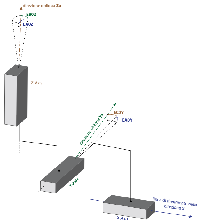
Fig.2 Un insieme di errori di orientamento rilevati in una macchina a 3 assi XYZ e utilizzati per la compensazione della sua ortogonalità
