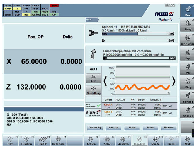
CNC NUM Flexium+ 8 con gestione sensore GAP
