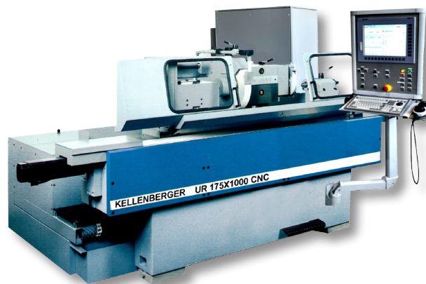
Revisione della macchina Kellenberger UR 175X1000 dal 2020
