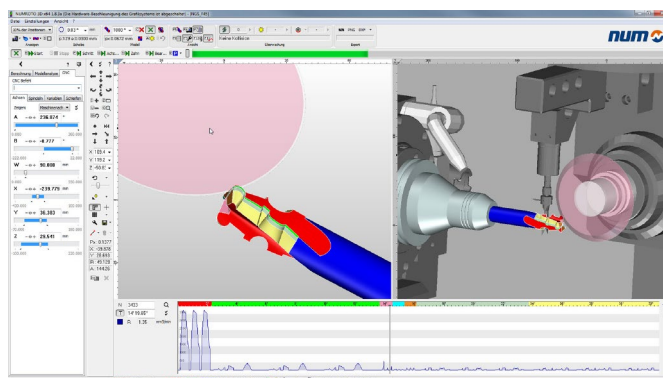
Esempio di simulazione NUMROTO 3D.
