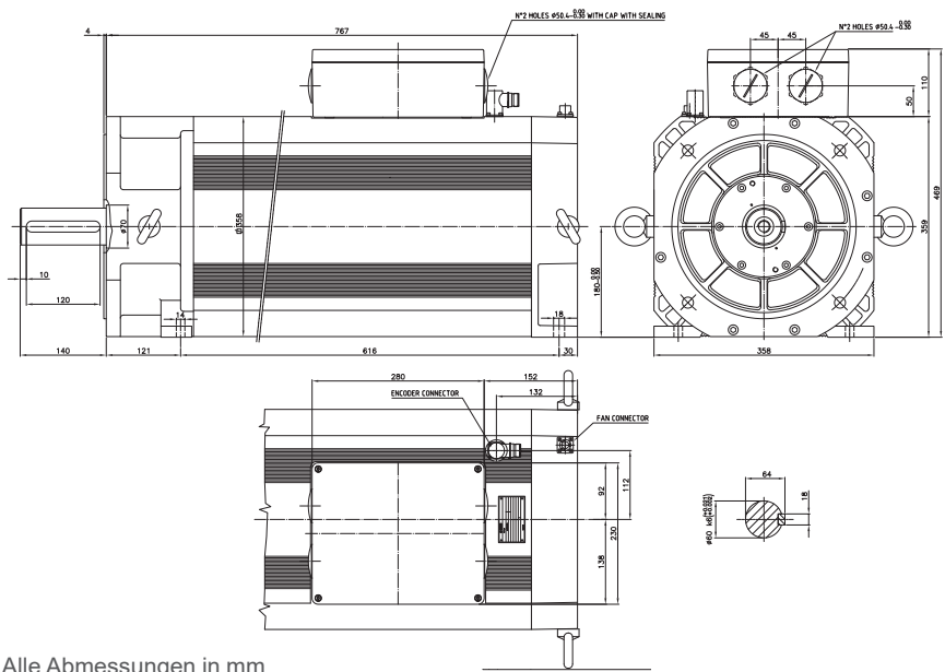
Motor IM 18MK14
