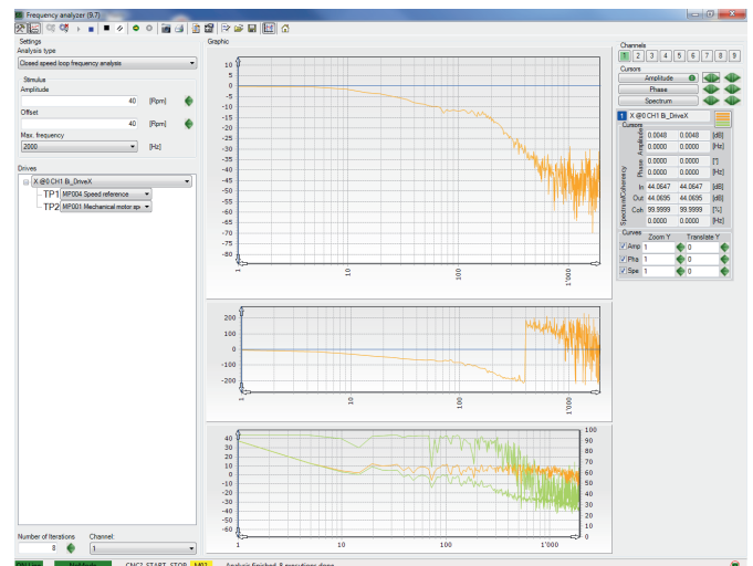
Beispiel eines Frequenzanalysator-Verfahrwegs
