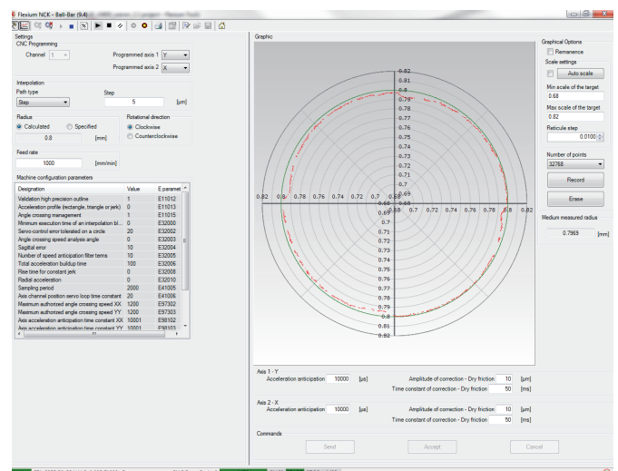
Beispiel eines Kreisformtest-Verfahrwegs
