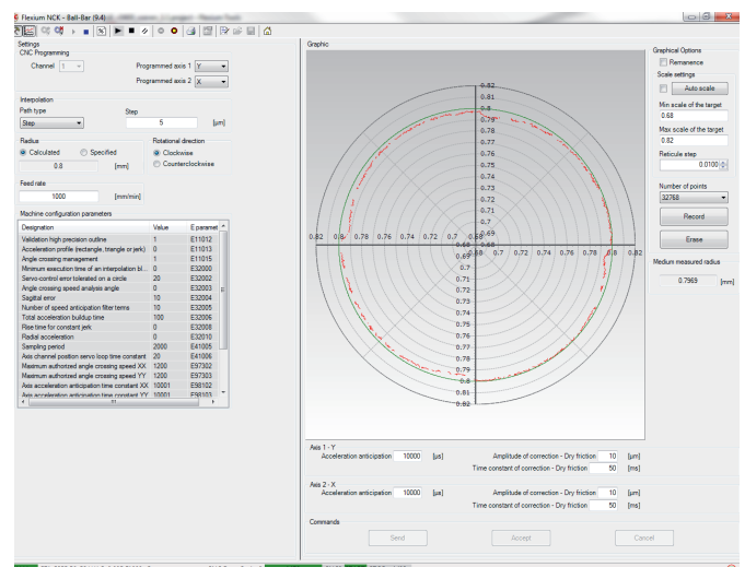
Beispiel eines Kreisformtest-Verfahrswegs
