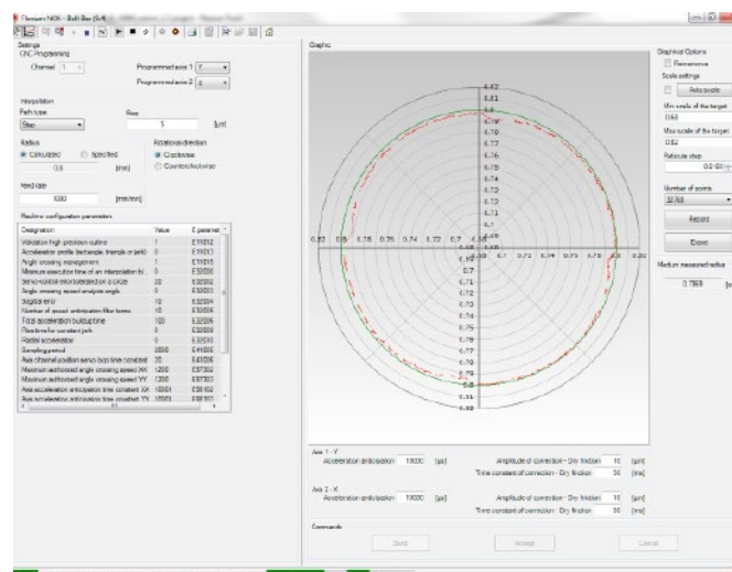
Exemple de trace ballbar
