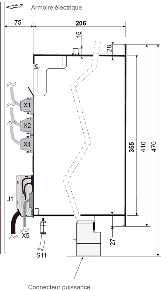
Dimensions des MDLUX et MDLL (taille 4)
