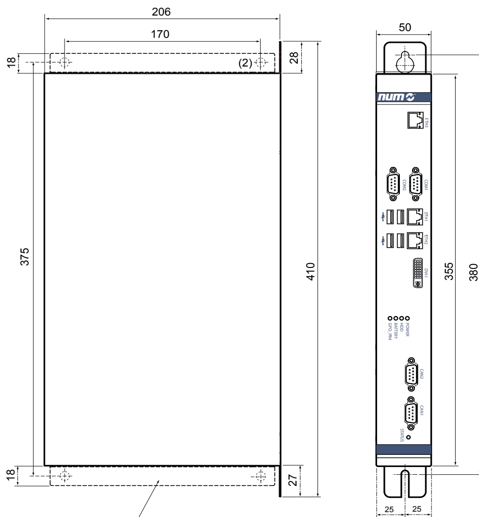
NUM 工業盒式 PC P1 簡圖 (FXPC004NN1SNR3A)
