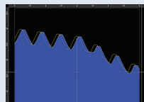
NUMROTO 2D 仿真详图 经过特殊计算的轮廓每个齿各不相同，并且在刀具的纵轴上也有偏移。
