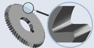
NUMROTO 中的 3D 仿真 高精度螺纹铣刀，附有高精度 3D 仿真的细节区域。刀具直径：50 毫米 -> 仿真精度 1 微米
