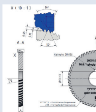
Extrait du dessin de la fraise mère
