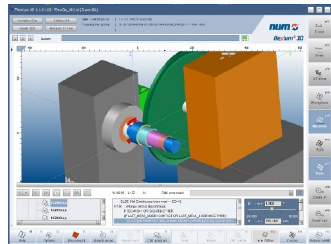
Vue complète de la simulation en ligne avec affichage des séquences, enlèvement de matière et détection de collision.
