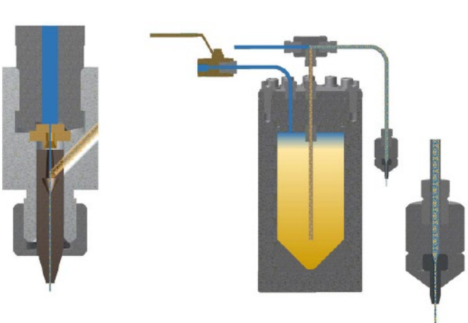
Dans la technologie par injection l'eau est introduite sous pression dans une chambre de mélange ce qui génère une dépression qui va aspirer l'abrasif. Dans la technique par suspension, l'eau et l'abrasif sont mélangés intimement puis l'ensemble est alors mis sous pression.
