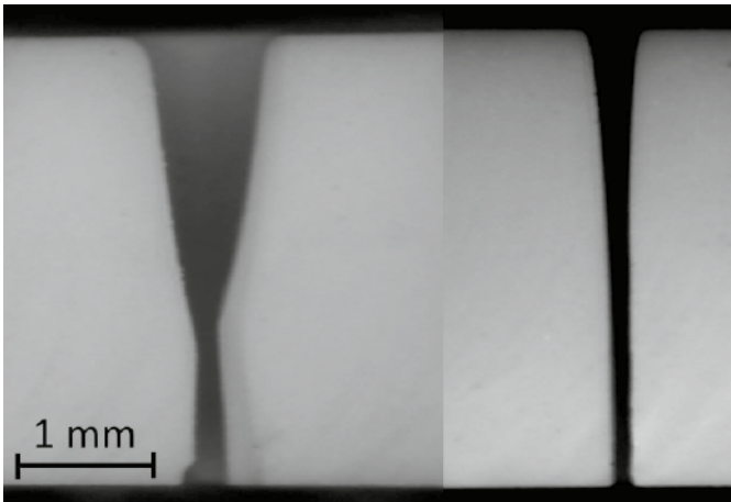
Comparaison des coupes en technologie par injection (à gauche) et par suspension (à droite) dans de l'oxyde d'aluminium et sous la même pression.
