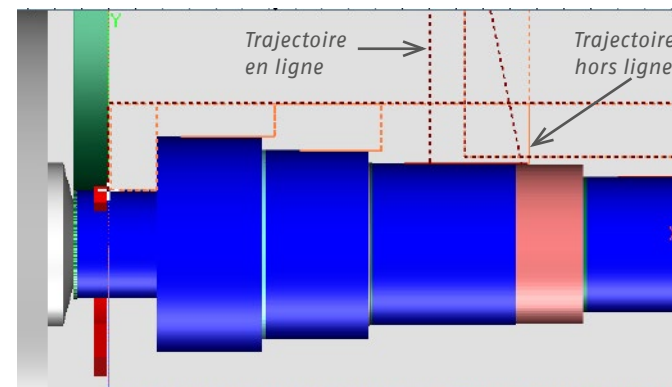
Vue complète de la simulation en ligne avec affichage des séquences, enlèvement de matière et détection de collision.
